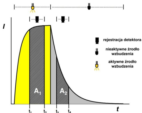
Rysunek 8. Schemat działania metody PDR. Po wzbudzeniu luminoforu, luminescencja jest rejestrowana za pomocą dwóch przedziałów czasu. Pierwszy jest umieszczony w fazie wzbudzenia ( A_1 ), drugi w fazie emisji ( A_2 ). Zmodyfikowano. [20]
